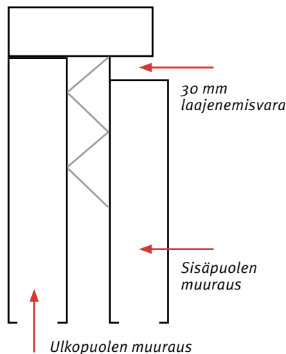
Ulko- ja sisäpuolen muurausta ei saa muurata kiinni toisiinsa, koska sisäpuolen lämpölaajeneminen on paljon suurempi kuin ulkopuolen. Mikäli ne muurataan kiinni toisiinsa, sisäpuolen lämpölaajene- minen rikkoo ulkopuolen muurauksen.
